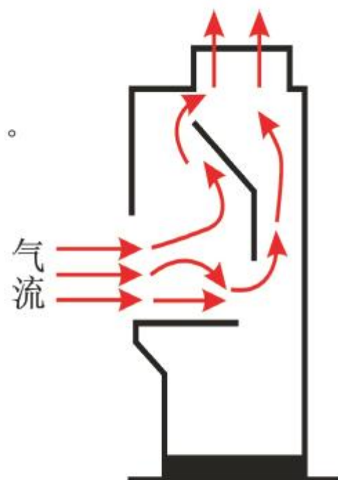
通风柜原通风原理
